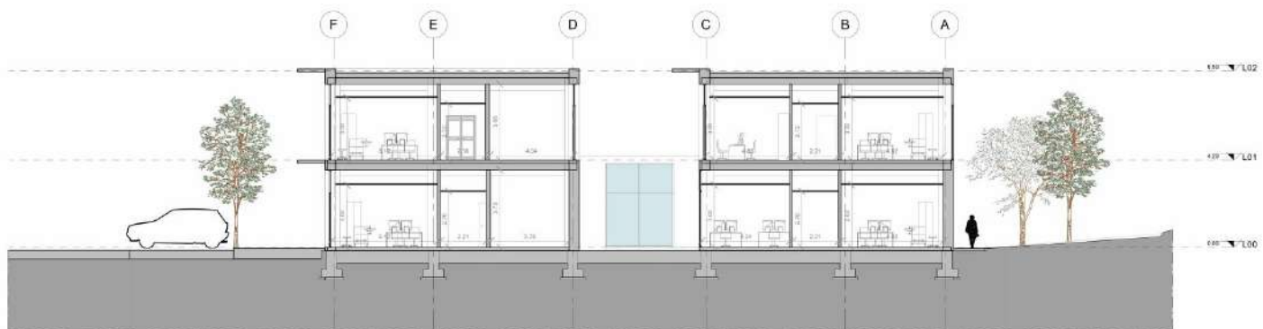
Sezione F-F 1:100
