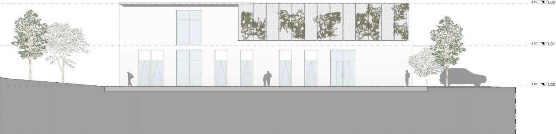
Prospetto Ovest 1 : 100
