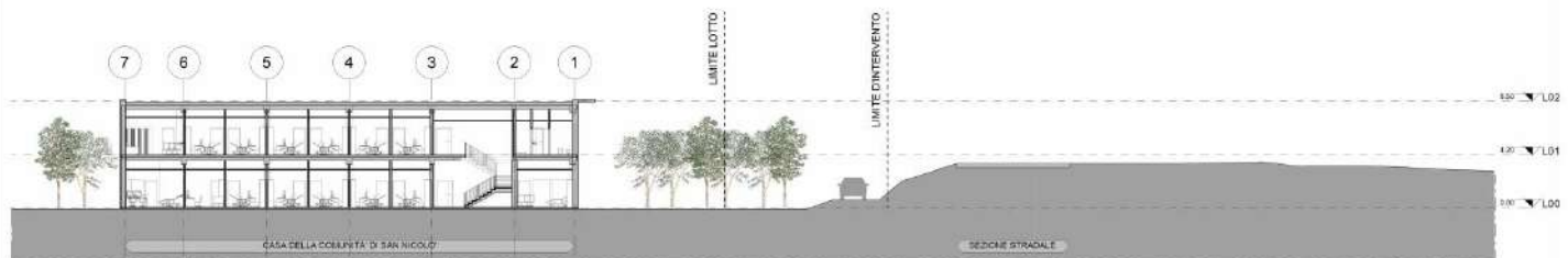
Sezione B-B 1 : 200
