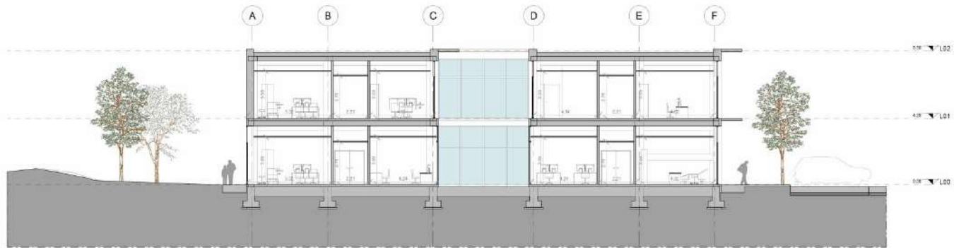
Sezione A-A 1 : 100
