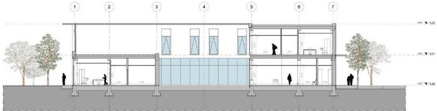
Sezione D-D 1:100
